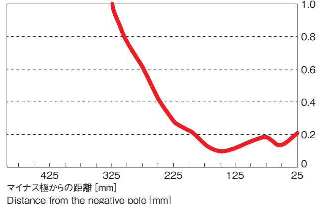
プラスに帯電した物体の除電時間 Removal Time for Positively Charged Object
