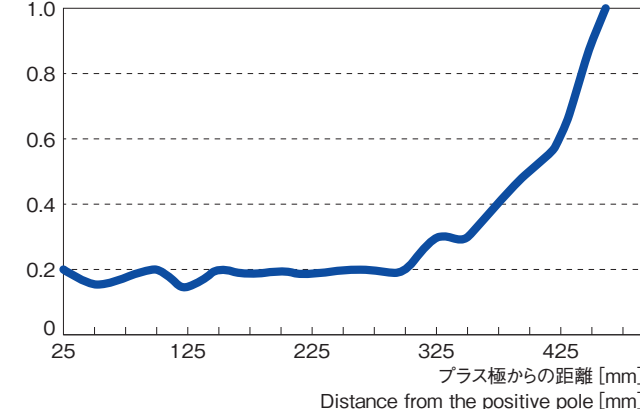
マイナスに帯電した物体の除電時間 Removal Time for Negatively Charged Object
